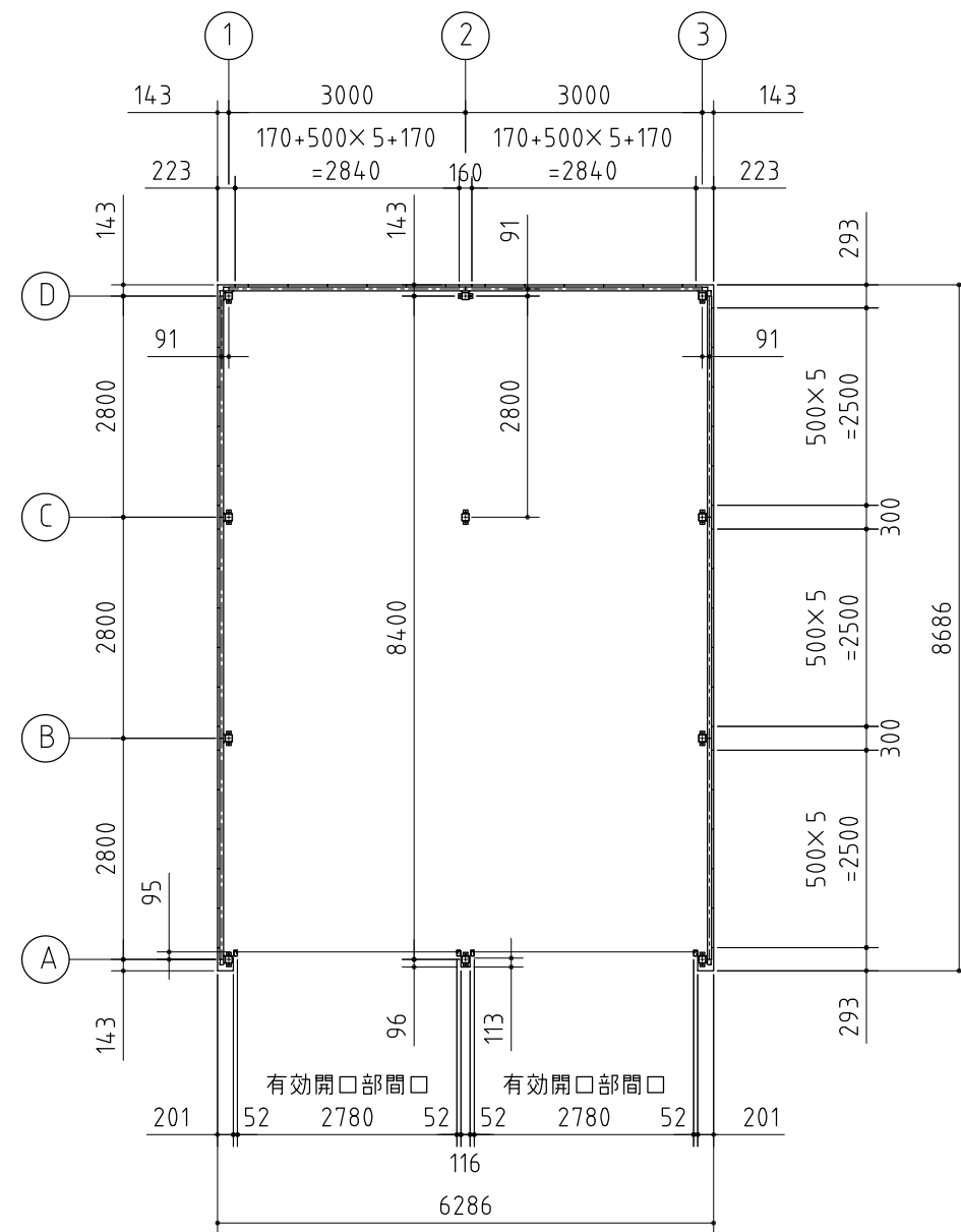
平面図
